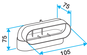
Verticaal bochtstuk 90°
