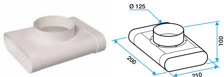
T-stuk onder een hoek van 90°, verticaal, voor ventiel
