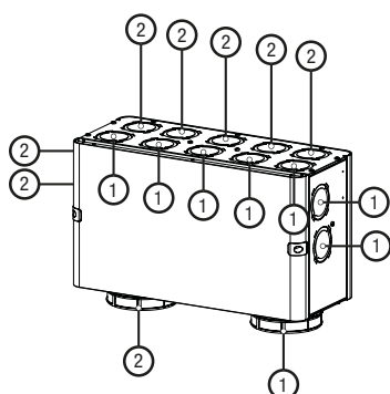
Schema voor de verdeling van de aansluitingen
