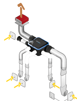
Installatie met MINIGAINE harde buizen
