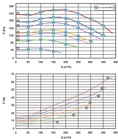
Ventilatie- en akoestische curve EasyHOME Hygro COMPACT SP
