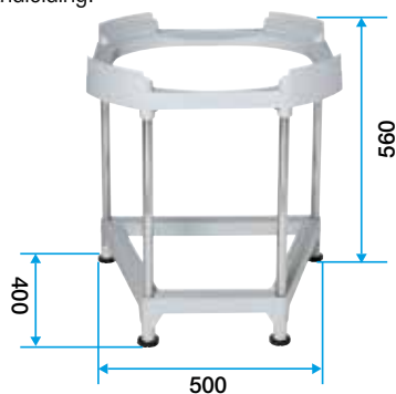
Buitenafmetingen van de T.Flow® Nano-sokkel
