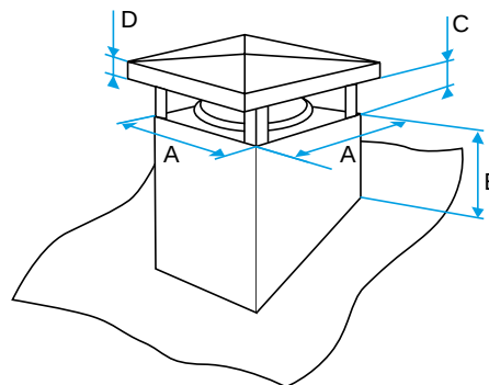
Maattekening Esthetische dakdoorvoer
