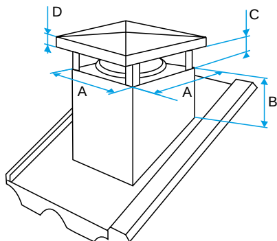
Maattekening Esthetische dakdoorvoer
