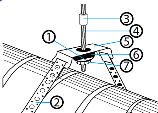
Montageschema van de montageband
