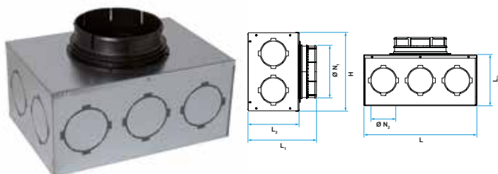
Caisson de répartition OPTIFLEX
