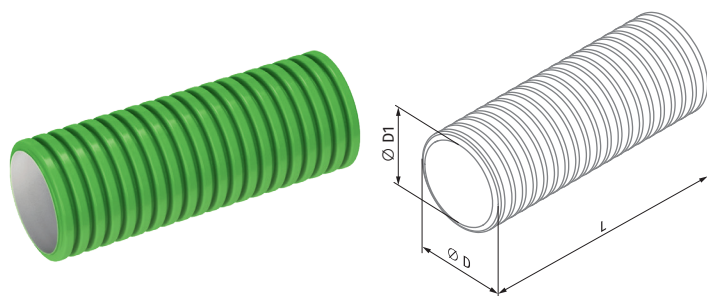
Ronde Optiflex®-buizen
