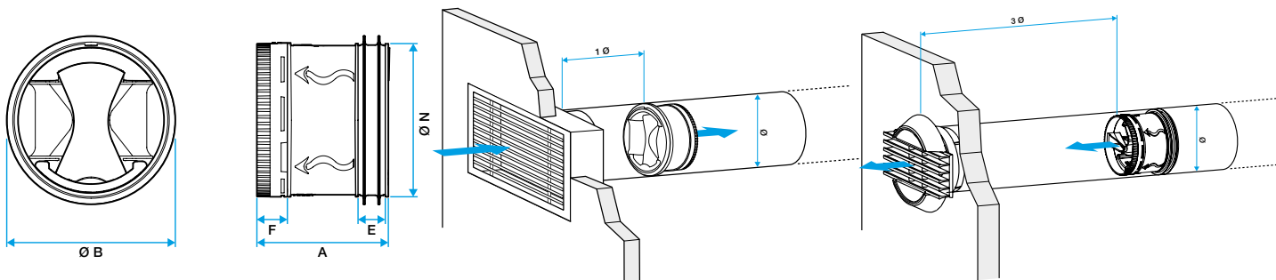
MR Modulo-afmetingen
