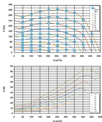
Aerailische en verbruikscurven en akoestische waarden EasyHOME SensAIR
