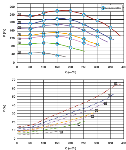
Aéraulische en akoestische curve EasyHOME Hygro COMPACT SP
