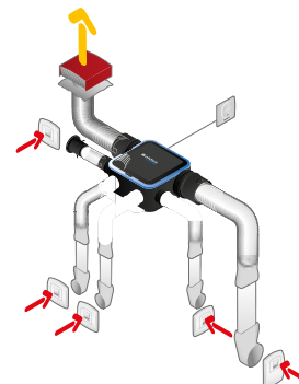
Installatie met MINIGAINE harde buizen
