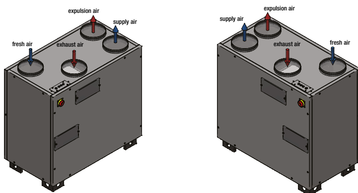
Oriëntatie van de luchtstromen InspirAIR® Top 1200
