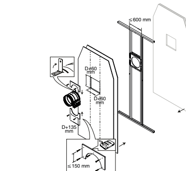
ISONE®2.1 circulaire sur cloison légère 120 minutes
