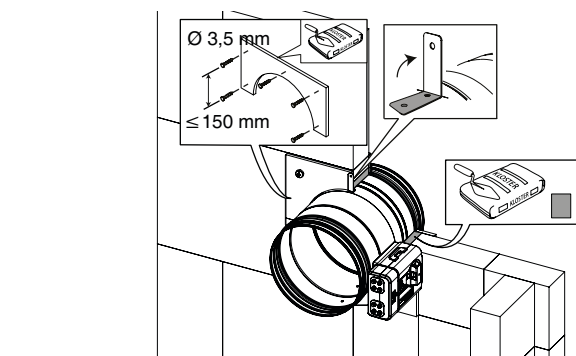
ISONE®2.1 circulaire sur cloison carreaux de plâtre 120 minutes
