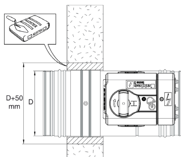
ISONE®2.1 circulaire sur mur béton
