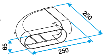
Horizontaal bochtstuk 90°
