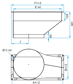
Rechthoekig > rond overgangsstuk VEX600
