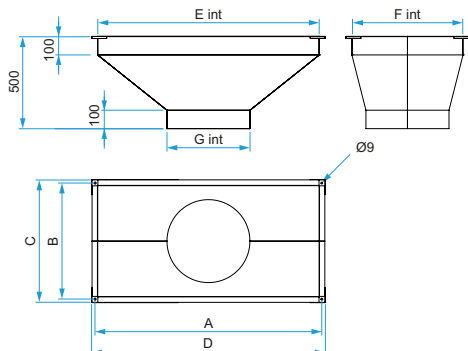
Rechthoekig > rond overgangsstuk VEX500
