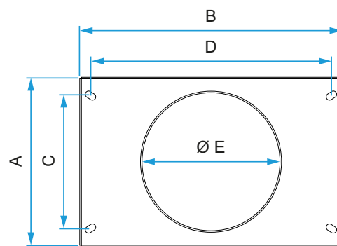
Rechthoekig > rond overgangsstuk VEX400
