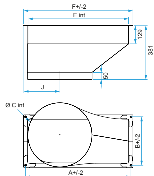
Rechthoekig > rond overgangsstuk VEX600
