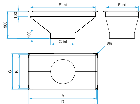
Rechthoekig &gt; rond overgangsstuk VEX500
