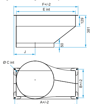
Rechthoekig &gt; rond overgangsstuk VEX600
