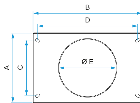
Rechthoekig &gt; rond overgangsstuk VEX400
