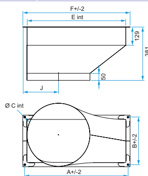
Rechthoekig &gt; rond overgangsstuk VEX600
