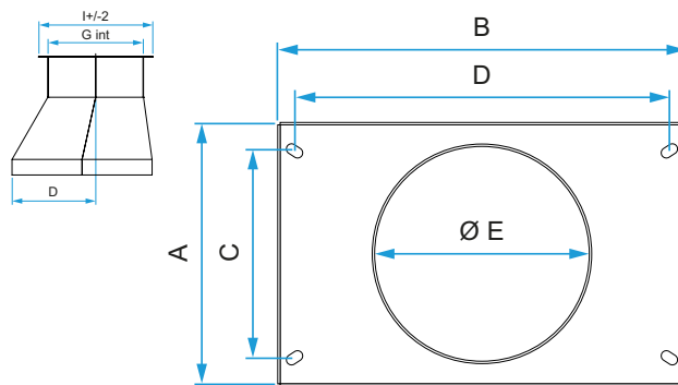
Rechthoekig &gt; rond overgangsstuk VEX400
