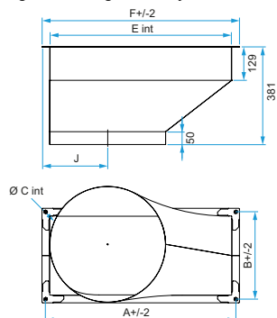
Rechthoekig &gt; rond overgangsstuk VEX600
