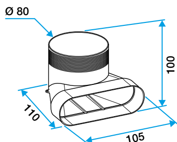
Gemengd bochtstuk voor ventiel met Ø 80 mm
