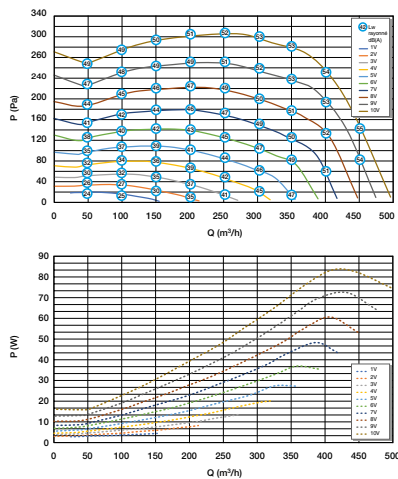
Aerologische en verbruikscurven en akoestische waarden EasyHOME SensAIR
