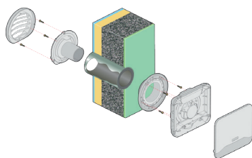
Composition entrée d'air EHT 2 et EFT 2
