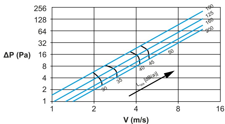
Drukverliescurve
