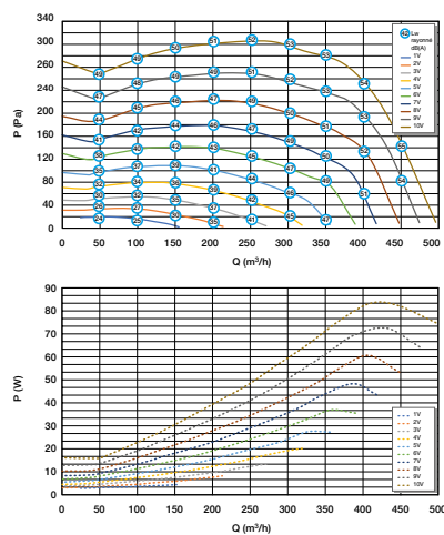
Aeraulische en verbruikscurven en akoestische waarden EasyHOME SensAIR
