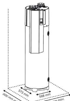
Installation de T.Flow® Hygro+ - Pose au sol
