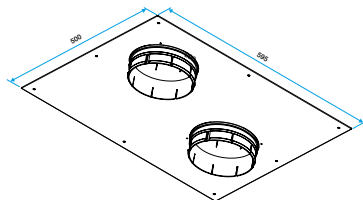
Plafondaafdichtingsplaat
