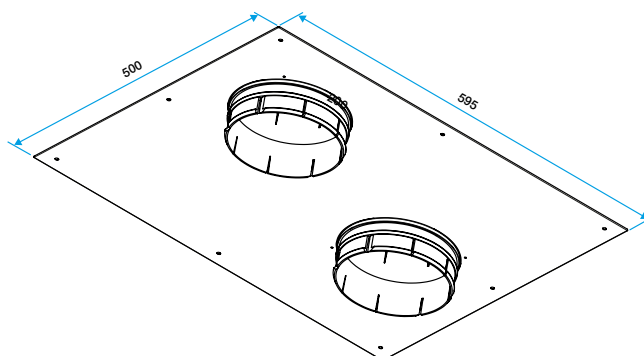
Buitenafmetingen plafondaafdichtingsplaat
