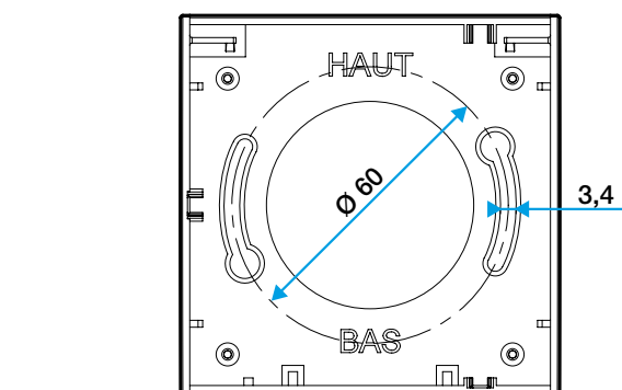
Dimensions C02 Mod (vue arrière)
