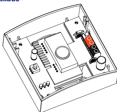
Câblage C02 Mod
