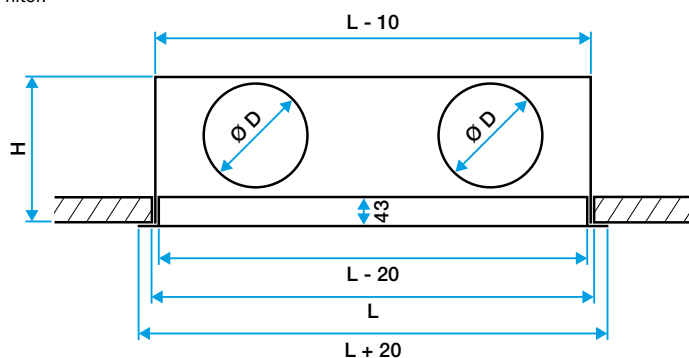
LINED-plenum
