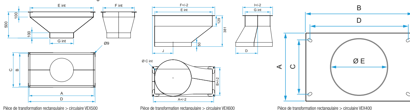
Pièce de transformation rectangulaire > circulaire VEX500
