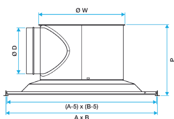
Diffuseur Twisted 850 pour dalles carrées
