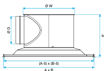
Diffuseur Twisted 850 pour dalles carrées
