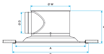
Diffuseur Twisted 850 pour plafond staff ou BA13
