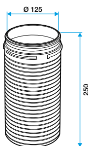
Rallonge circulaire Ø125 mm
