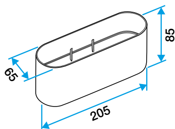
Raccord femelle 60x200 mm
