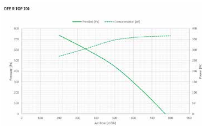
Courbe aéraulique DFE R TOP 700
