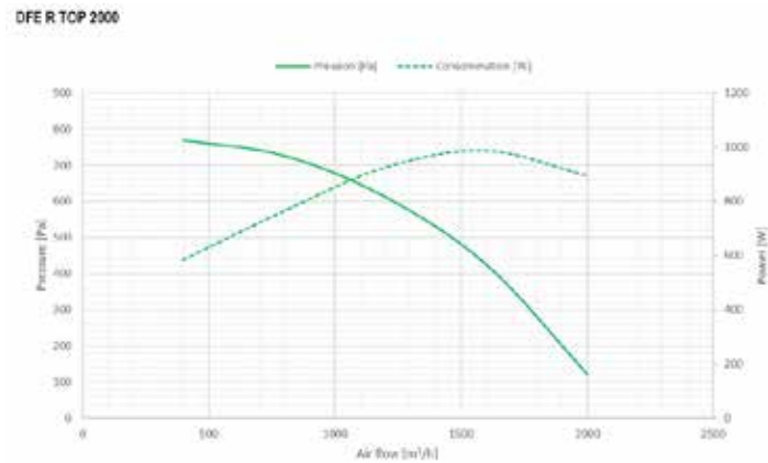
Courbe aéraulique DFE R TOP 2000
