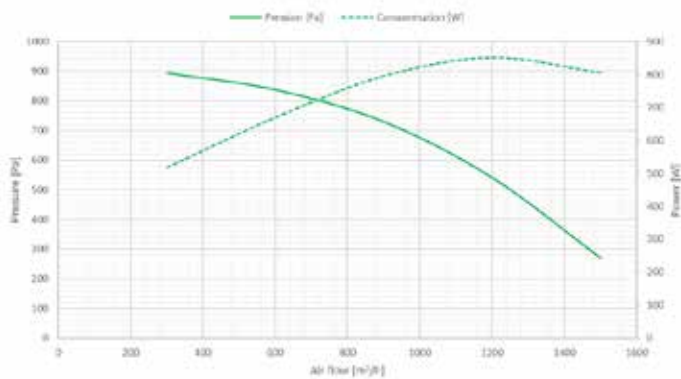
Courbe aéraulique DFE R TOP 1500
