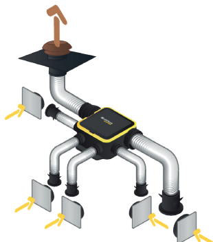
Installation kit Auto DHU COMPACT + ColorLINE avec conduits souples Algaïne
