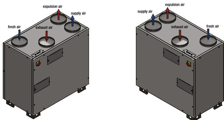
Orientation des flux d'air InspirAIR® Top 1200
