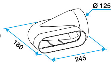
Coude 90° horizontal pour conduit
