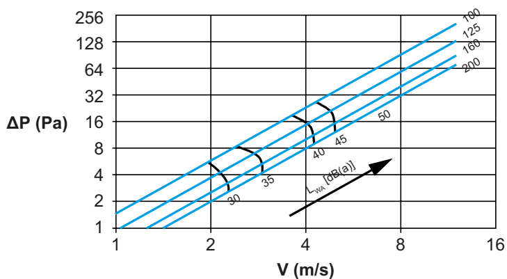
Courbe pertes de charge
