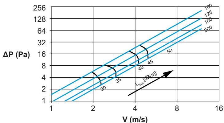
Courbe perte de charge
