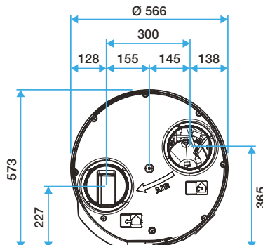
Encombrement T.Flow® Hygro+ - Raccordement aéraluque
