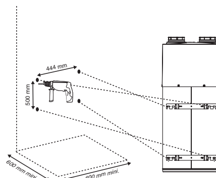
Installation de T.Flow® Nano - Installation au mur
