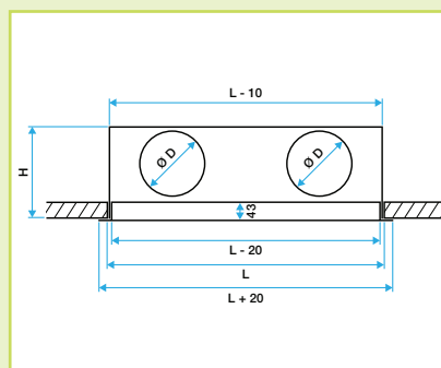
Rooster met bevestiging S2 of S3
