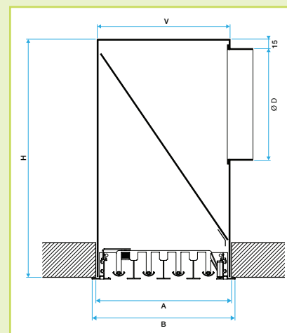
Afzuigrooster met plenum, bevestiging S2 en filter
