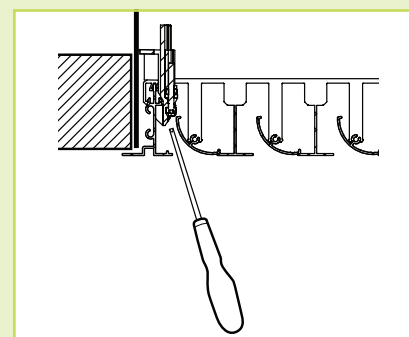
Verstelling bevestiging S3
