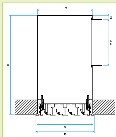
Uitblaasrooster met plenum, bevestiging S3
