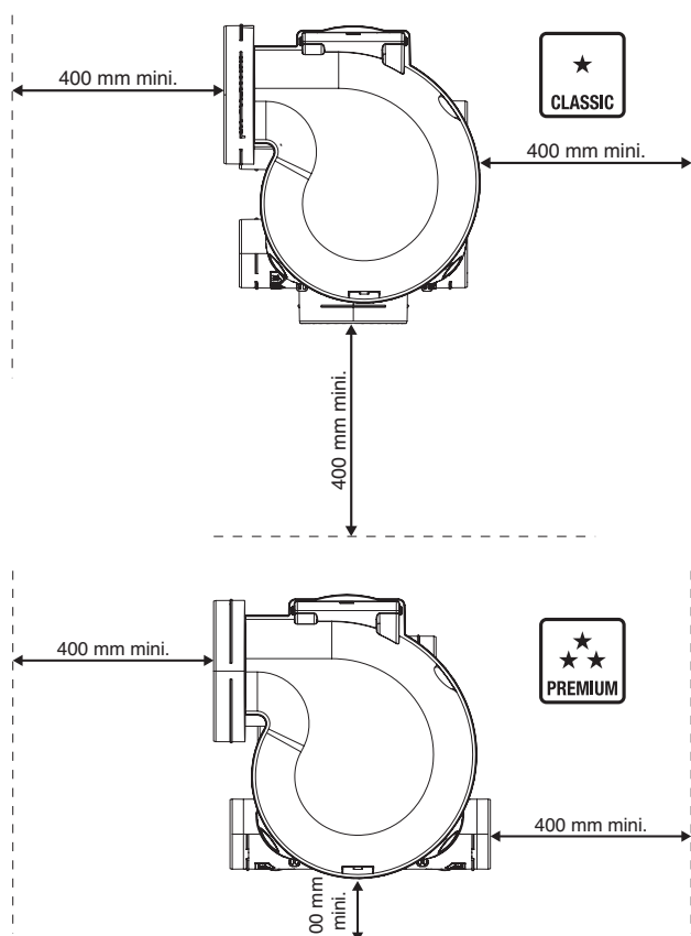
Bovenaanzicht
