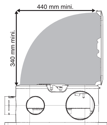
Zijaanzicht
