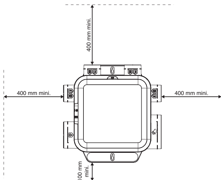
Bovenaanzicht
