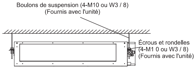
Illus. 3.4 L'installation de l'unité intérieure
