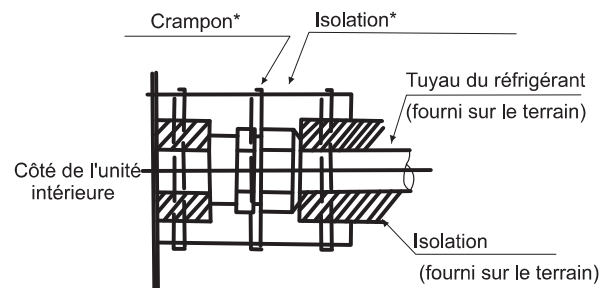
Illus. 4.4 Procédure d'isolation de la tuyauterie
