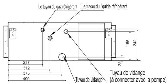
Illus. 4.1 Les positions de connexion du tube
