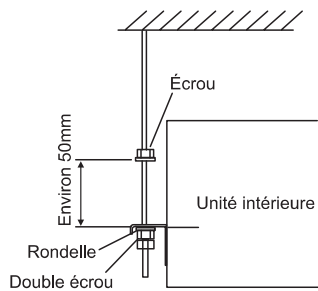
Illus. 3.5 Boulons de suspension et écrous
