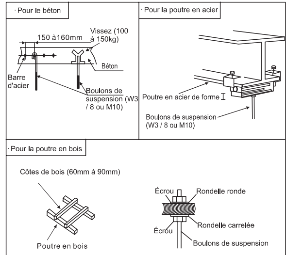
Illus. 3.2.1 Fixation des boulons de suspension
