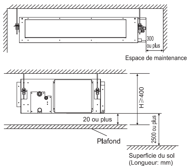
Illus. 3.1.2 (Unité : mm)
